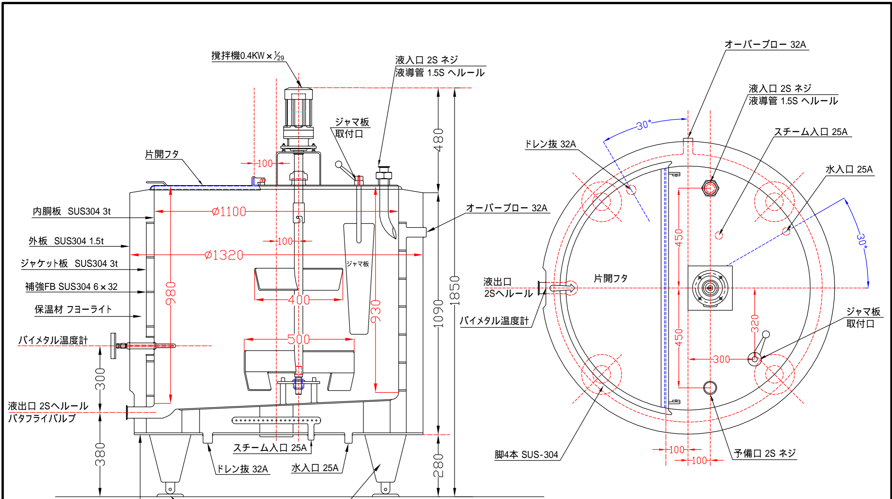
殿 800 加熱冷却タンク
